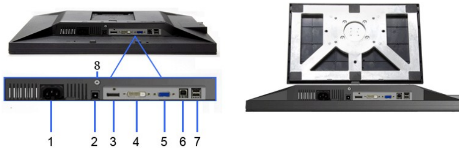
底面部
